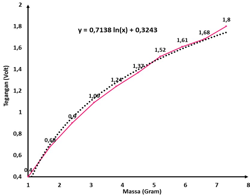
Gambar 7. Grafik hasil karakterisasi tegangan keluaran sensor strain gauge yang dirangkai jembatan Wheatsone beserta penguat diferensial terhadap penambahan beban massa dengan kelipatan 0,7 gram dengan span antara 1 gram sampai 7,3 gram.
