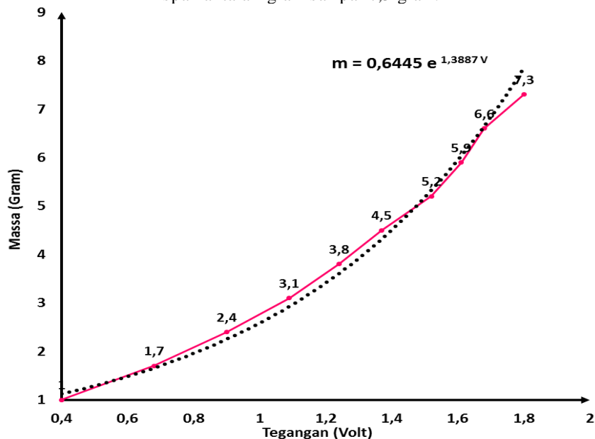
Gambar 7. Grafik hasil karakterisasi tegangan keluaran sensor strain gauge yang dirangkai jembatan Wheatsone beserta penguat diferensial terhadap penambahan beban massa dengan kelipatan 0,7 gram dengan span antara 1 gram sampai 7,3 gram.
