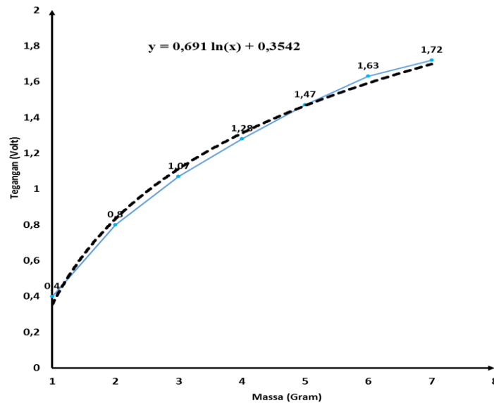
Gambar 5. Grafik hasil karakterisasi tegangan keluaran sensor strain gauge yang dirangkai jembatan Wheatsone beserta penguat diferensial terhadap penambahan beban massa dengan kelipatan 1 gram dengan span antara 1 gram sampai 7 gram.
