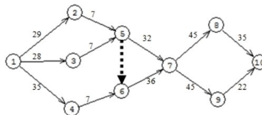
Gambar 1. Visualisasi digraf jalur truk
