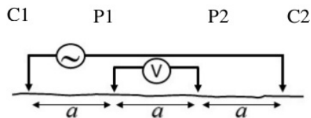
Gambar 2. Konfigurasi Wenner
