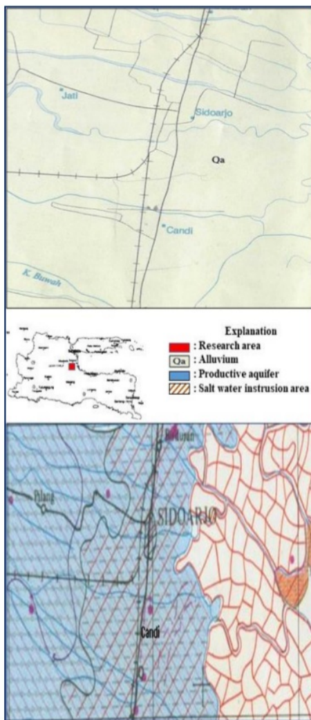
Gambar 1. Kondisi geologi dan hidrogeologi
