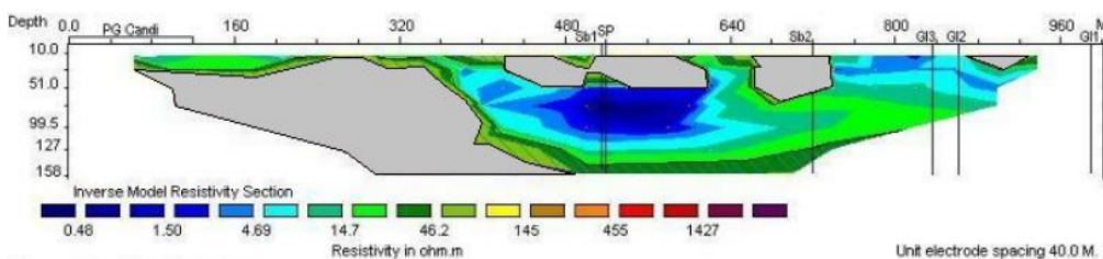
Gambar 5. Sebaran akuifer air asin dan air tawar
