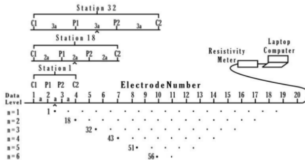
Gambar 3. Desain survei 2D konfigurasi Wenner (Loke, 2013)
