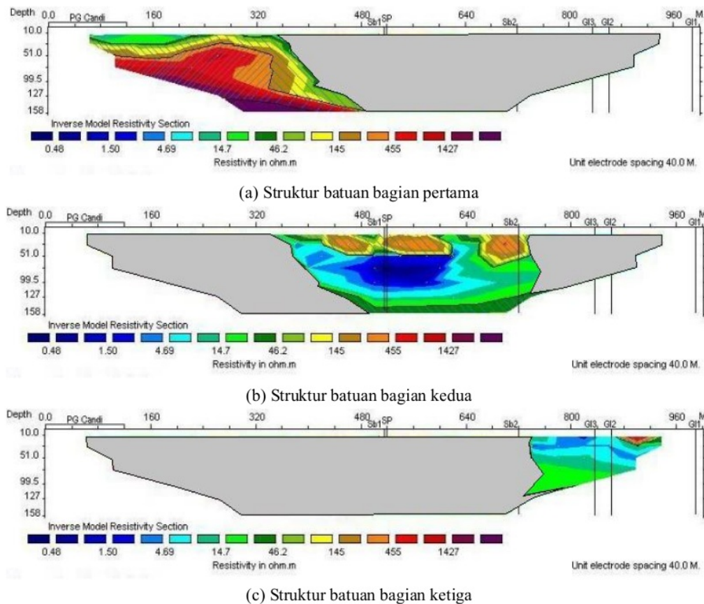
Gambar 4. Struktur batuan bawah permukaan
