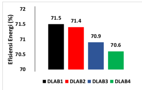
Gambar 6 Efisiensi baterai DLAB dengan berbagai macam variasi luas permukaan
