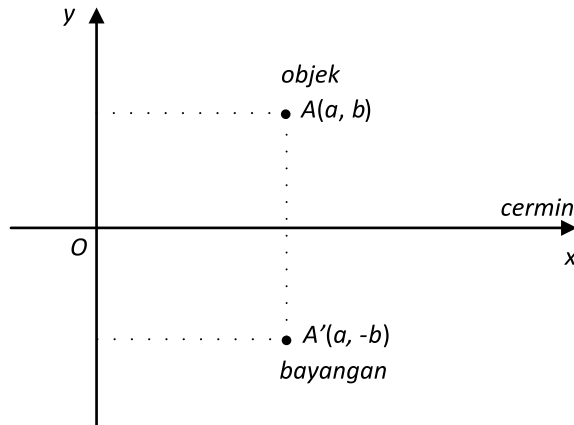
Gambar 10.9 Pencerminan terhadap sumbu x
