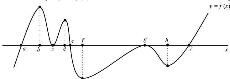
Gambar 11.18 Sketsa turunan pertama suatu fungsi y = f(x)
