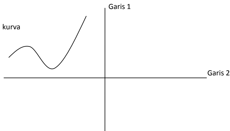
Gambar 10.6 Pencermianan kurva oleh cermin garis 1 dan garis 2
