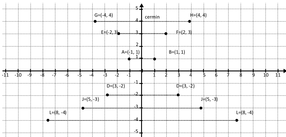
Gambar 10.11 Pencerminan titik terhadap sumbu y
