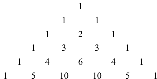
Diagram di atas dikenal dengan sebutan segitiga Pascal
