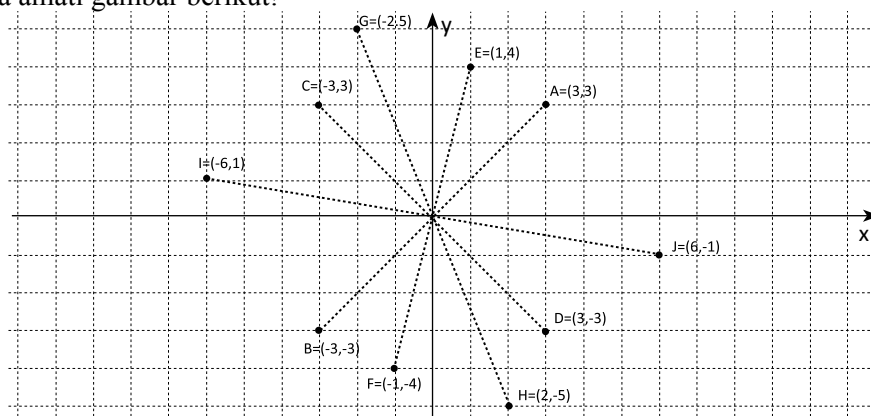
Gambar 10.7 Pencermianan terhadap titik asal koordinat
