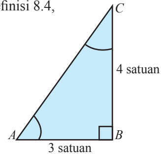
Gambar 8.10 Segitiga siku-siku
