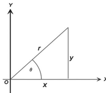
Gambar 8.25 Segitiga siku-siku
