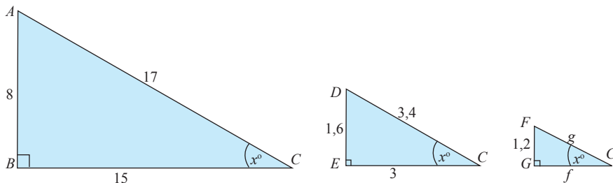
Gambar 8.9 Kesebangunan
