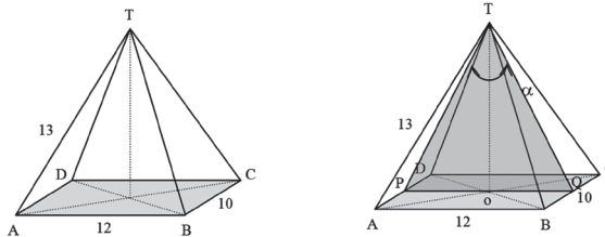
Gambar 9.46 Limas T.ABCD
