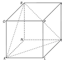
Gambar 9.23 Kubus KLMN.OPQR
