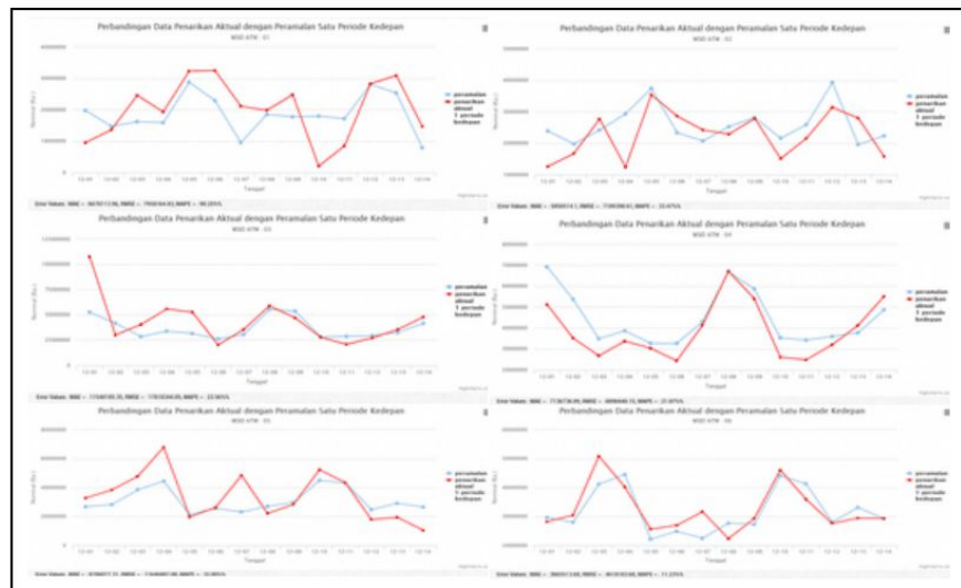
Gambar 12 Grafik penarikan aktual dan peramalan satu periode kedepan pada bulan Desember berdasarkan pengujian bulan Januari hingga bulan November
