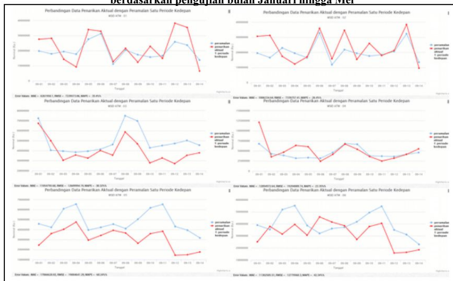
Gambar 11 Grafik penarikan aktual dan peramalan satu periode kedepan pada bulan September berdasarkan pengujian bulan Januari hingga Agustus
