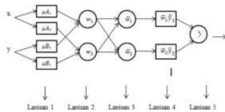
Gambar 2.1 Arsitektur Jaringan ANFIS
